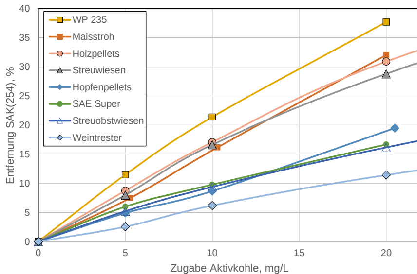
Abbildung 9: Entfernungslleistung verschiedener CoAct-Kohlen bezüglich SAK(254)
