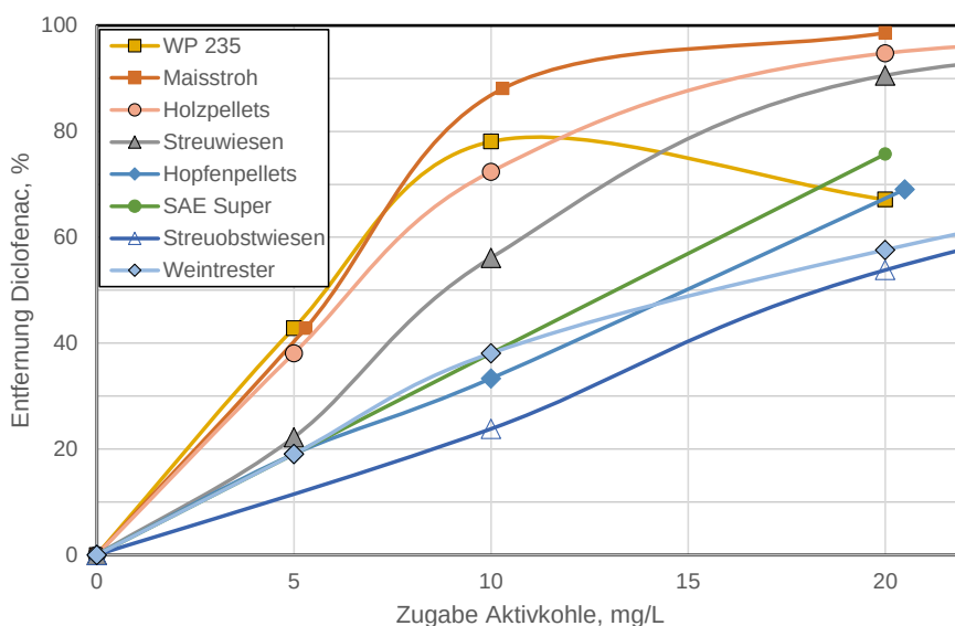
Abbildung 10: Entfernungslleistung verschiedener CoAct-Kohlen für Diclofenac
